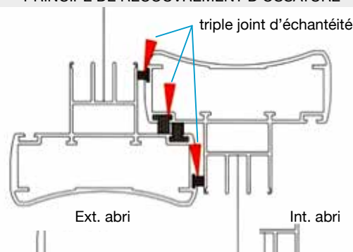
PRINCIPE DE RECOUVREMENT D'OSSATURE
